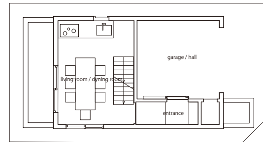
1F Plan S=1/150
